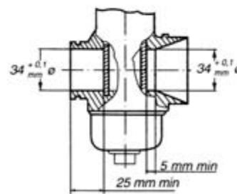
CARBURETTOR SECTION PRZEKRÓJ GAŹNIKA
