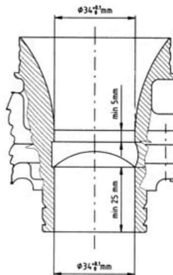
CARBURETTOR SECTION PRZEKRÓJ GAŹNIKA
